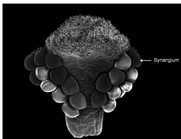
Abb. 9 & 10: Zamia amblyphyllidia , Detail eines Mikrosporophylls, adaxial (links) und abaxial (rechts); auf der abaxialen Seite stehen die Mikrosporangien zu dritt in kurz gestielten Synangien vereint;
